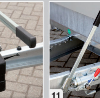
5-stufiger, sehr starker Zylinder, Kippwinkel 48° (bis 6100 kg)
